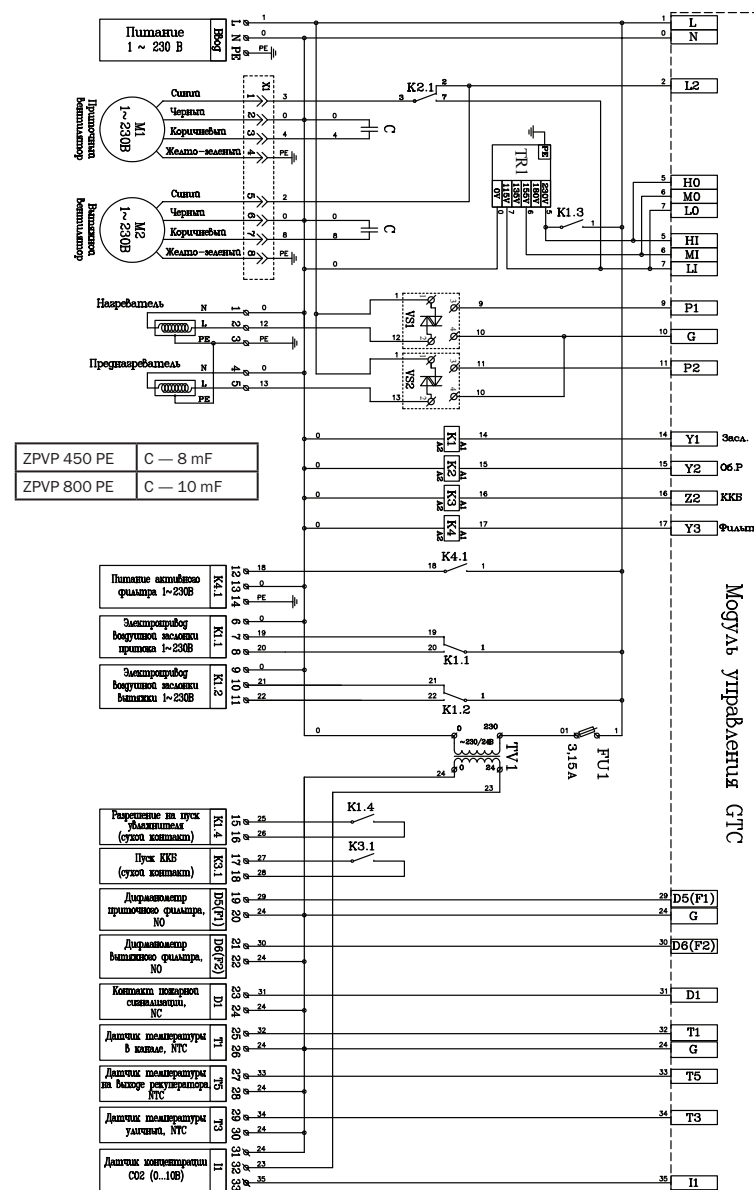
Схема автоматики ZPVP 450 PE, ZPVP 800 PE
