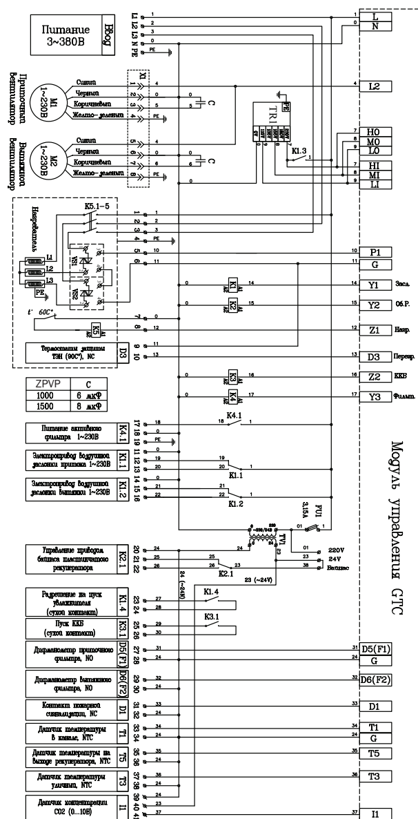
Схема автоматики ZPVP 1000 PE, ZPVP 1500 PE
