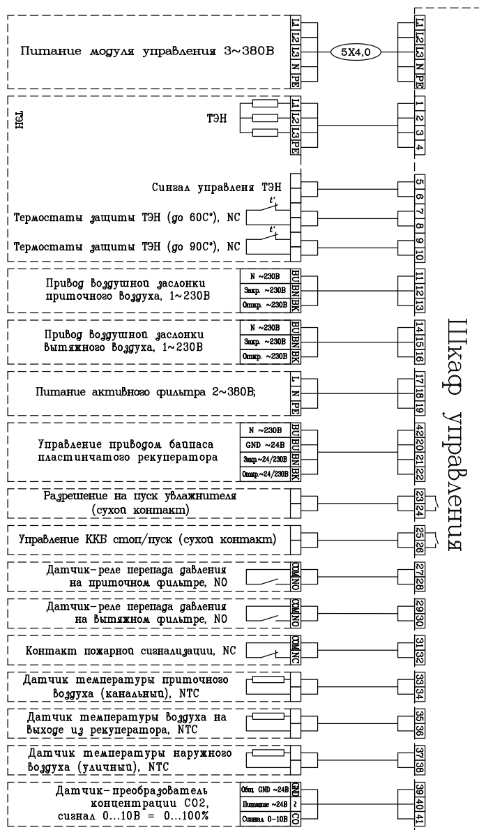
Схема подключения ZPVP 1000 PE, ZPVP 1500 PE
