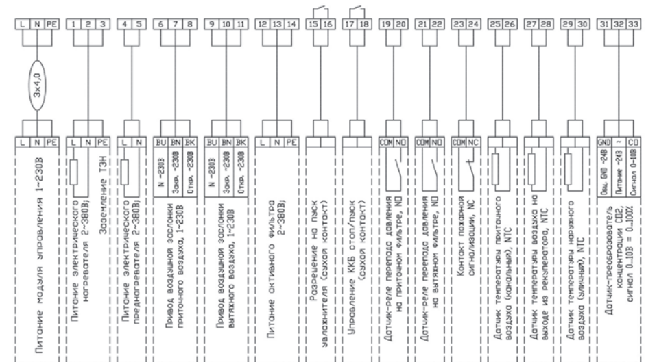
Схема подключения ZPVP 450 PE, ZPVP 800 PE
